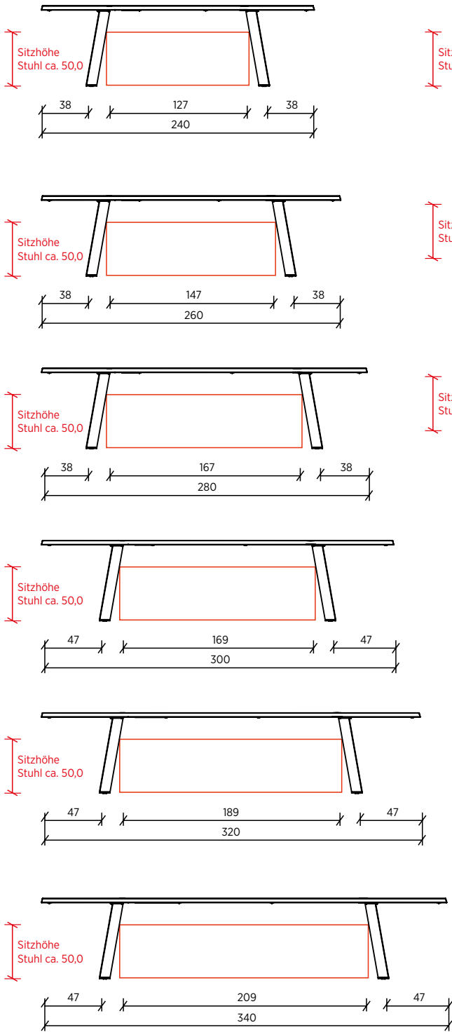
Abbildung: längsseitig
