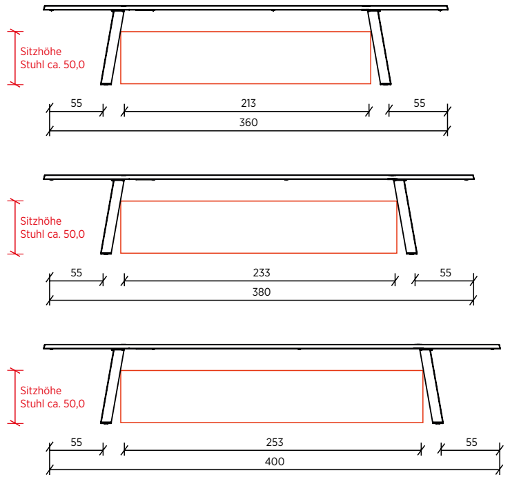
Abbildung: längsseitig
