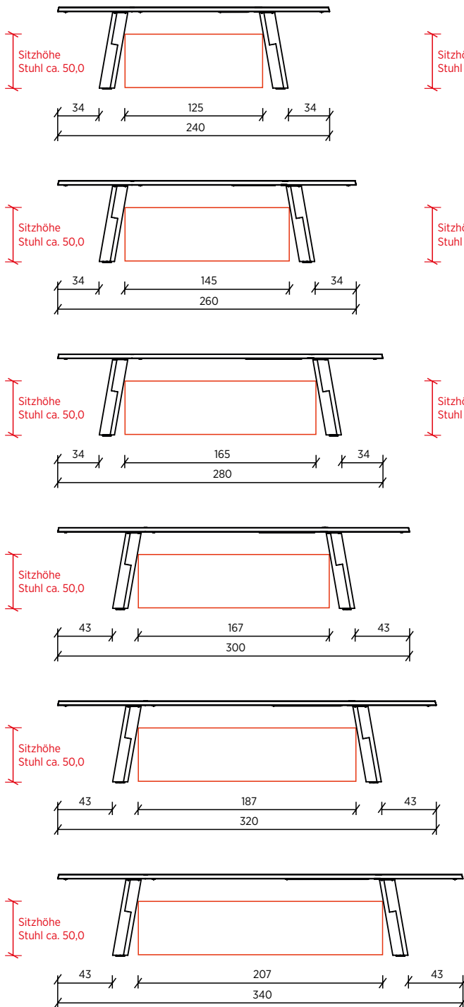
Abbildung: längsseitig
