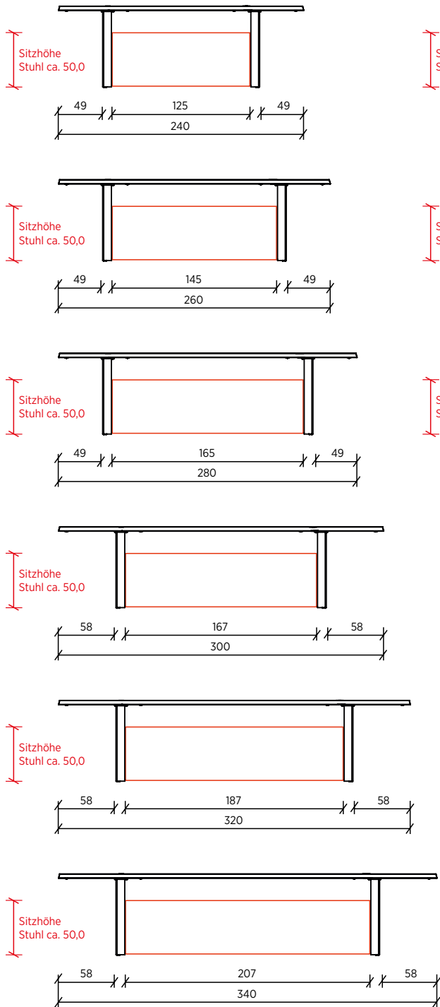
Abbildung: längsseitig
