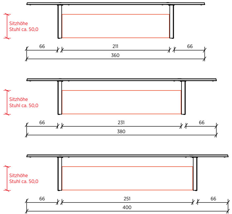
Abbildung: längsseitig
