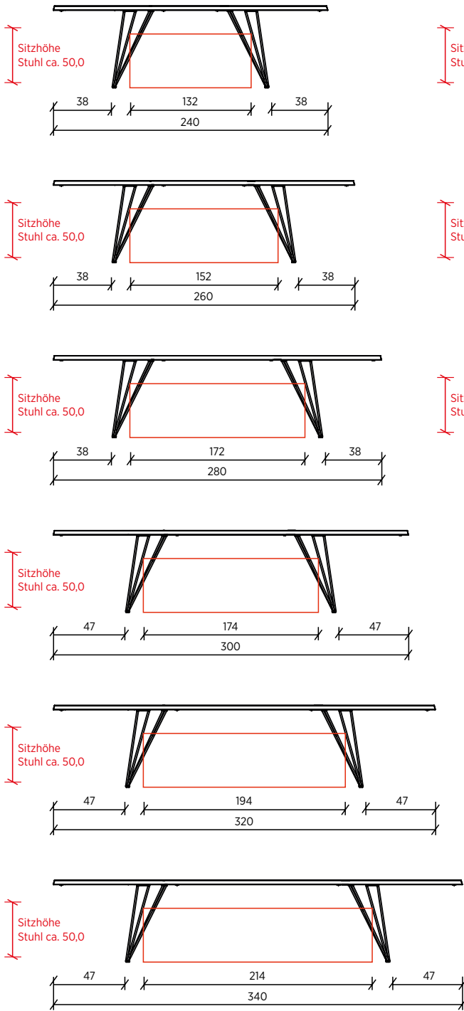
Abbildung: längsseitig
